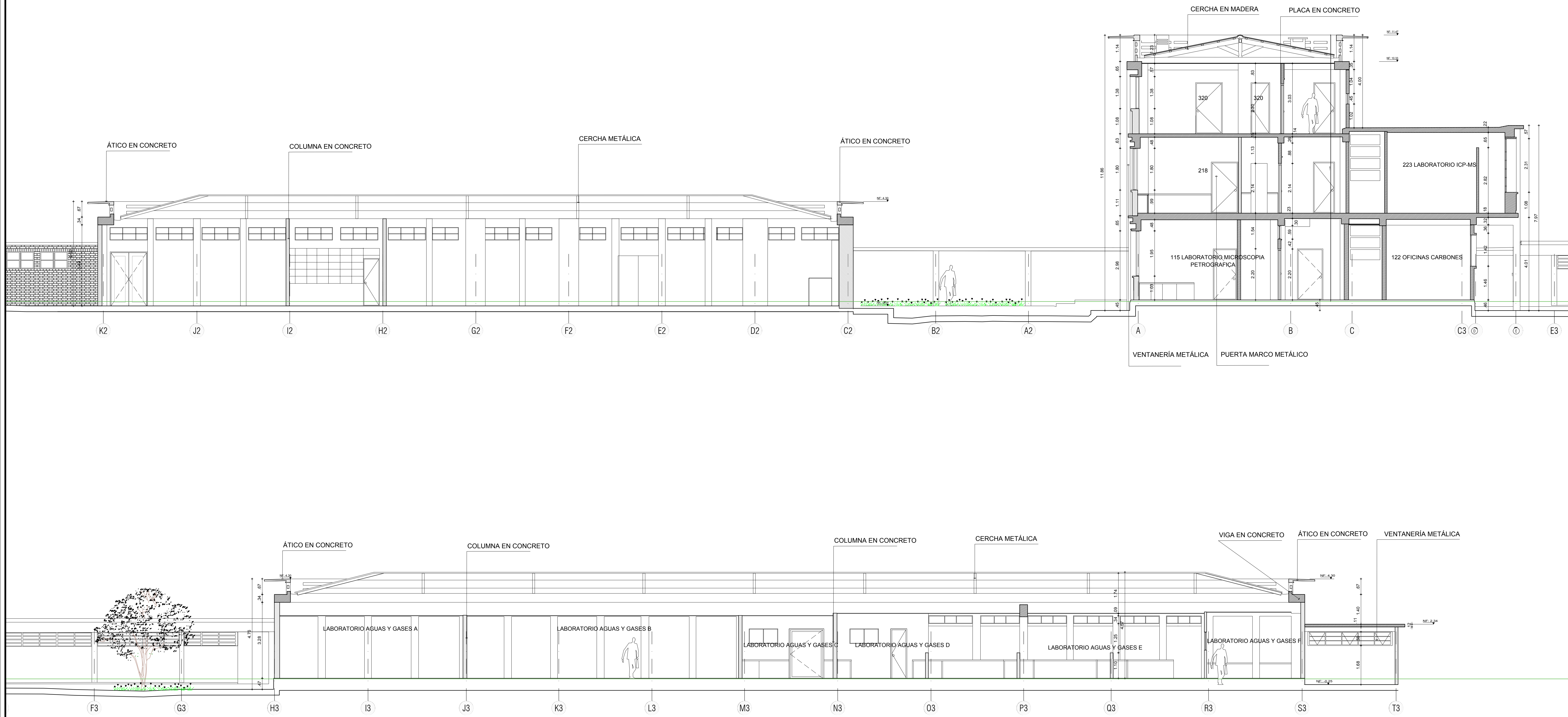
CORTE ACT-01 ESCALA 1:75
